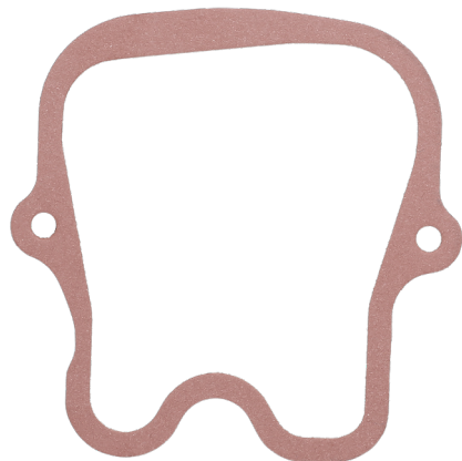
Vecchia 638.901 – MAN 51.03905.0134 Materiale: EWP rosso (materiale morbido)
